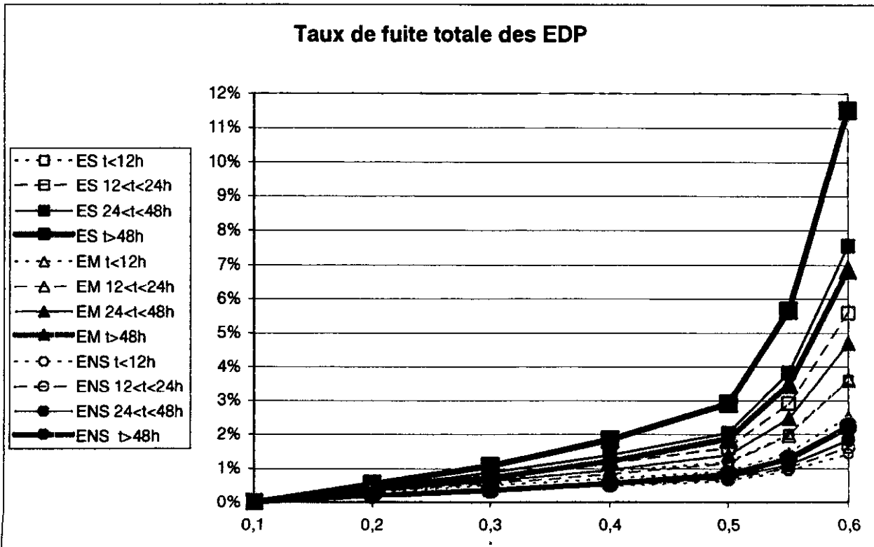
Graphique 4.7.b : Taux de fuite totale des EDP
