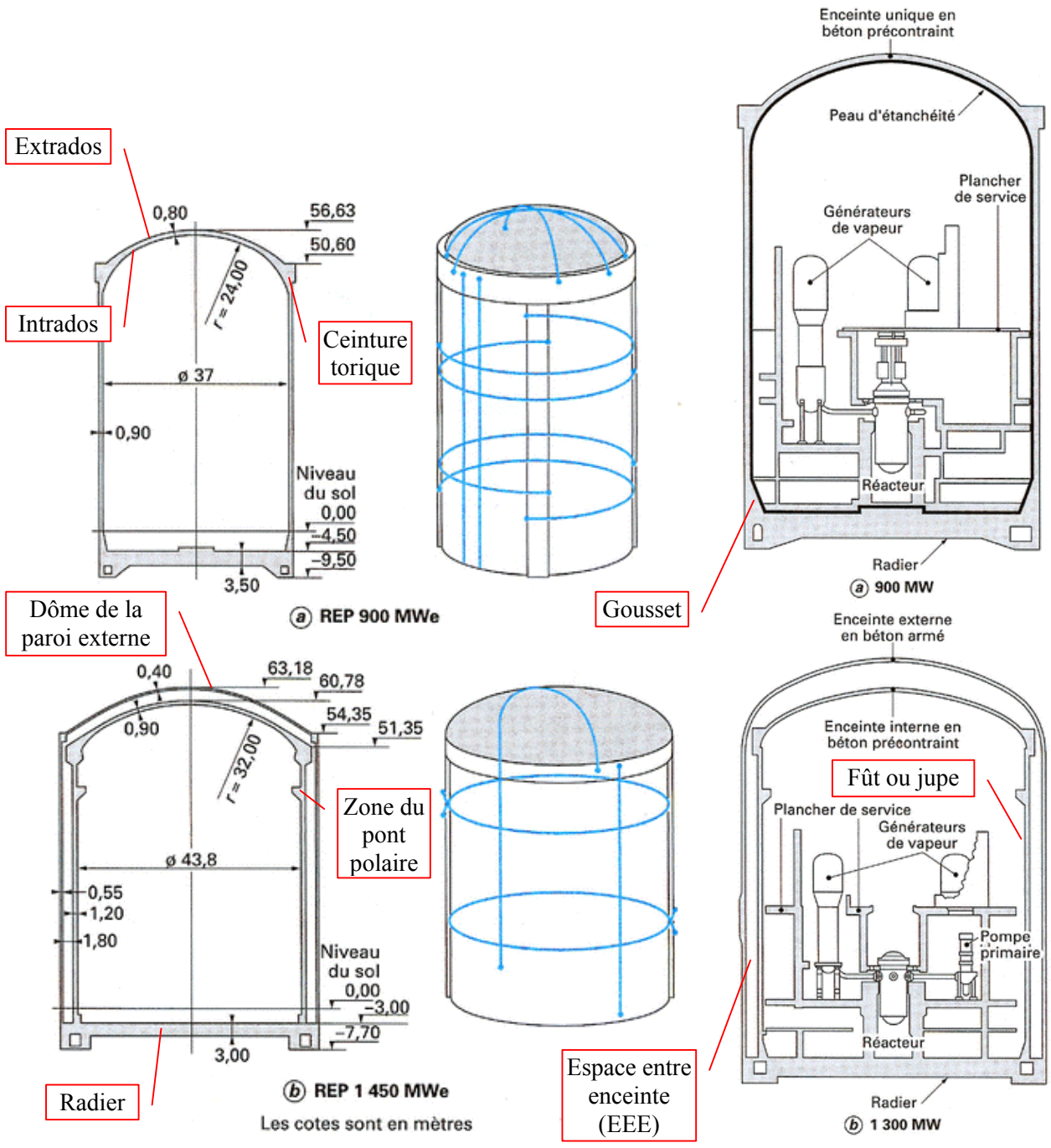
Principales dimensions et tracé de la précontrainte
